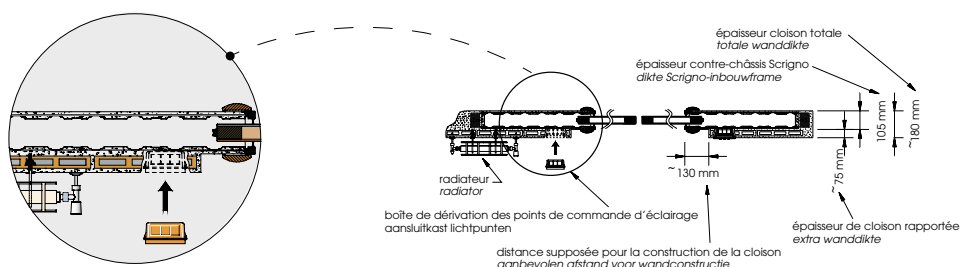
Détail: logement de la boîte de dérivation Detail: inbouwen van de aansluitkast
