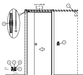
Exemple d'installation sur une porte existante Voorbeeld installatie op bestaande frame
