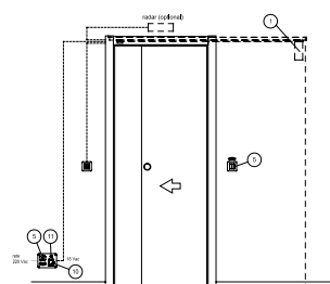
Exemple d'installation sur une nouvelle porte Voorbeeld installatie op nieuwe frame
